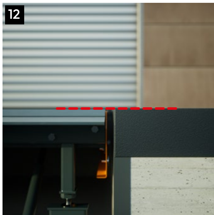
Sollevare tutta la rampa dall'ancoraggio anteriore (compreso) finché il pianale non è in piano con la banchina / Lift the entire ramp, including the front anchorage, until the deck is level with the dock.
