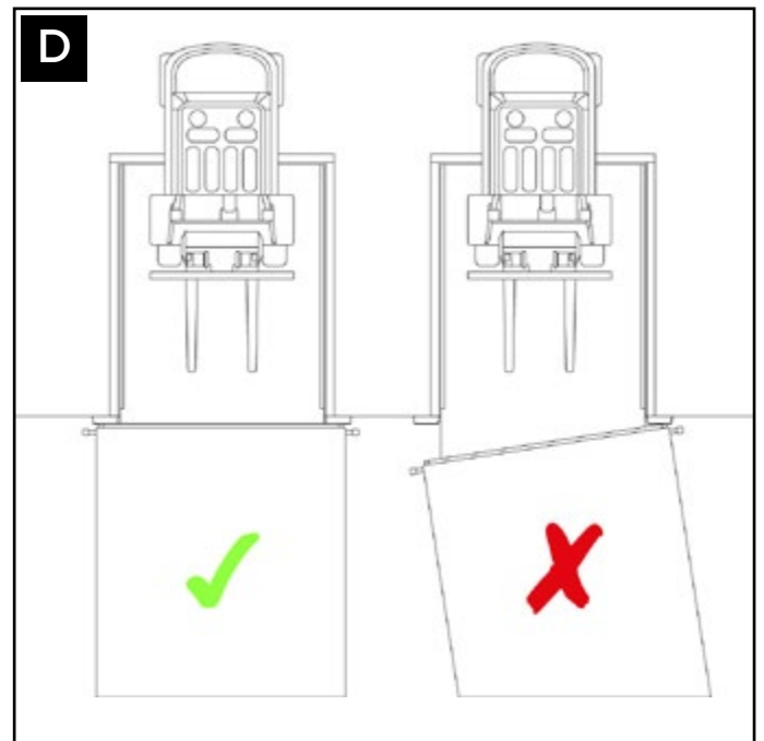
Transitare unicamente quando la pedana è ortogonale / Start work only when the truck is in a orthogonal position
