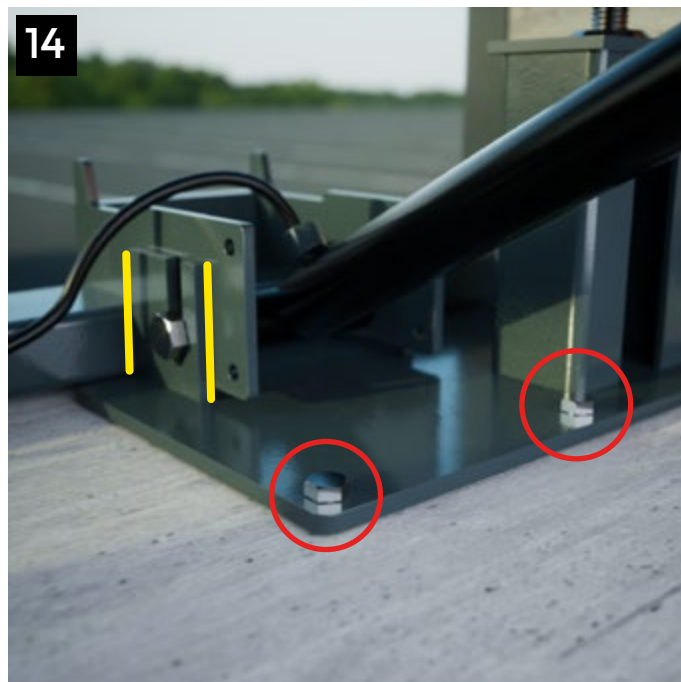
Regolare le due piastre di appoggio dell'ancoraggio anteriore e tassellarle sul fondo della fossa per poi saldare da entrambi i lati come indicato in figura / Adjust the two support plates of the front anchorage and anchor them to the bottom of the pit then weld on both sides as shown in the figure.
