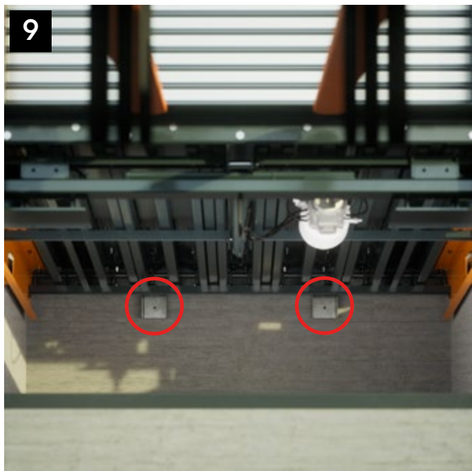
Tassellare l'ancoraggio posteriore alla parete della fossa / Anchor the rear anchorage to the pit wall using anchors.
