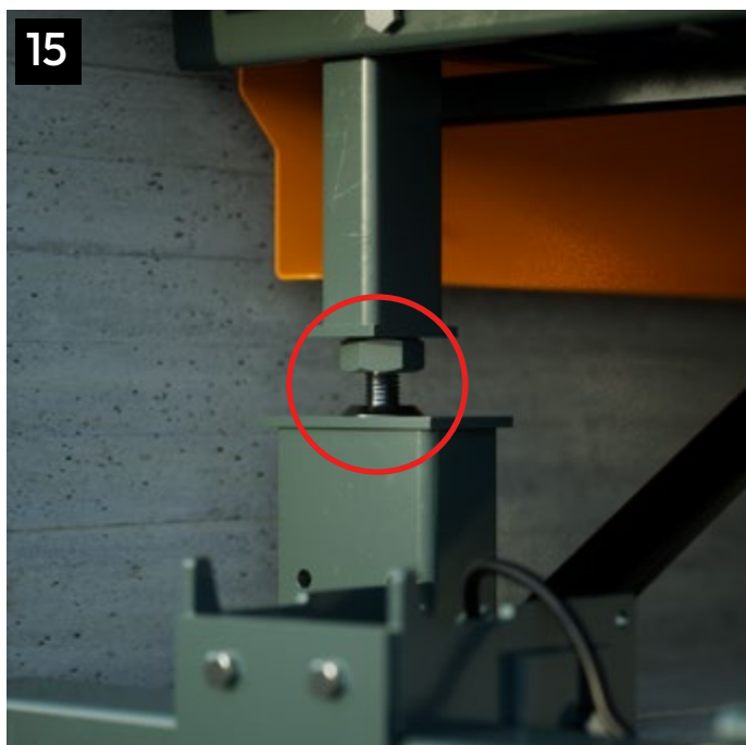
Se necessario regolare la quota pianale con il piedino di appoggio / If necessary, adjust the platform height using the support foot.
