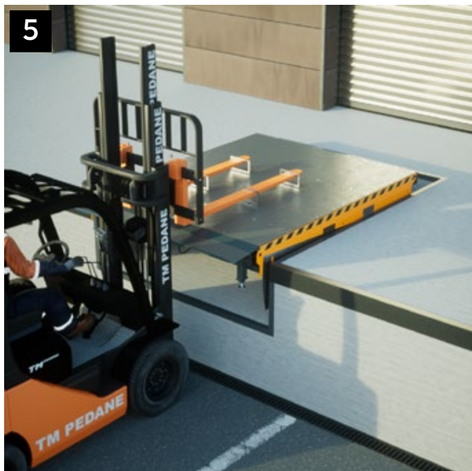
5 Inserire con cautela la rampa nella fossa / Carefully insert the ramp into the pit.
