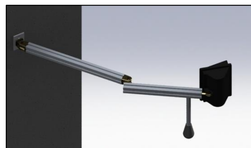
Braccetto in alluminio estruso con snodi in acciaio zincato e sistema d'illuminazione a 500W
